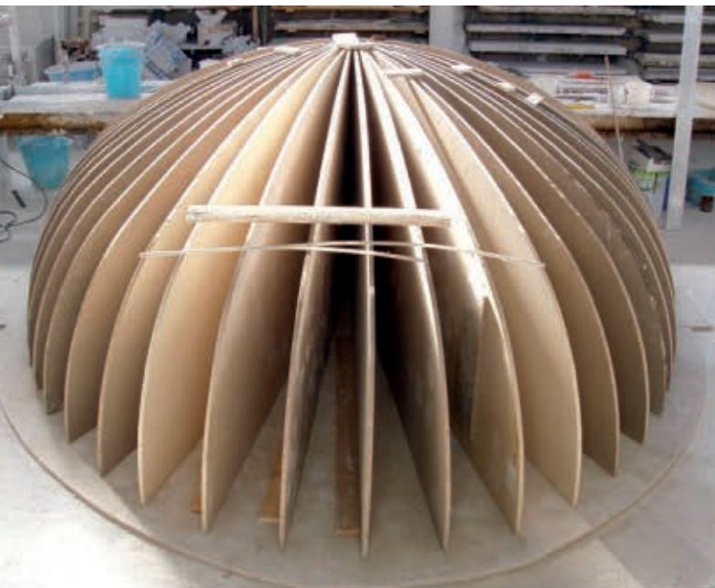
Realizzazione di una cupola ovale ellittica / Creation of an elliptical oval dome
